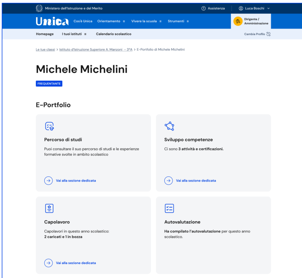
FIGURA 27 –SCHERMATA E-PORTFOLIO/AUTOVALUTAZIONE
